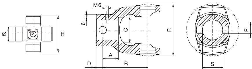
圆孔刀具万向节叉和注滑脂附件
