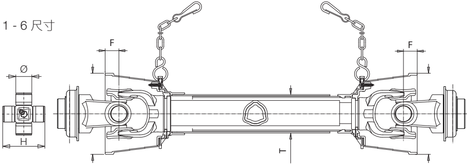
G9 尺寸
