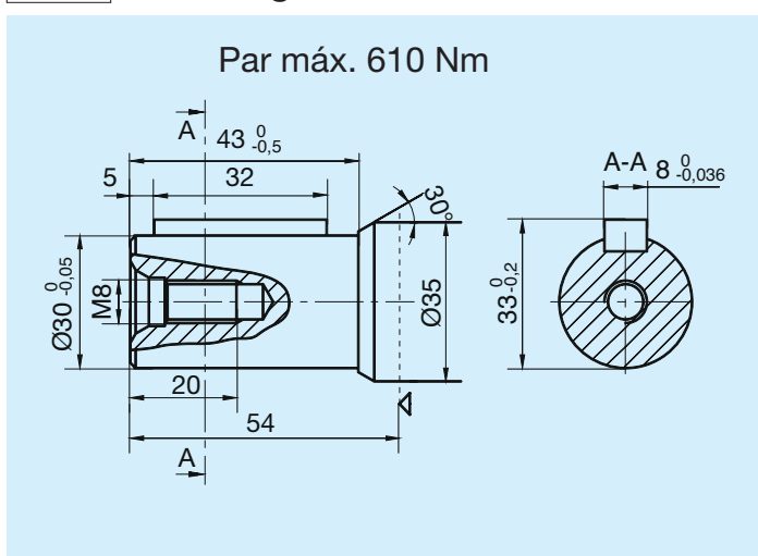
AP2 Ø30 lengüeta DIN 6885 A 8x7x32
