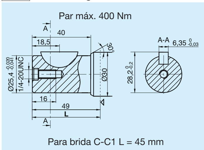
AP4 1" USA lengüeta BS46 1 1/4"
