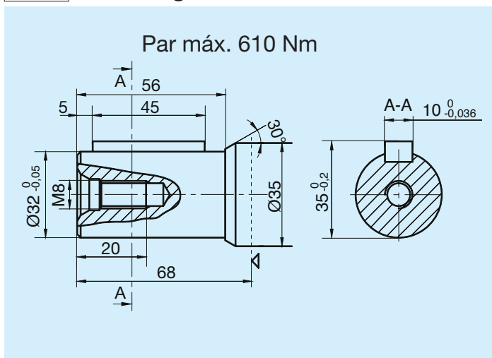
P52 Ø32 lengüeta DIN 6885 A 10x8x45
