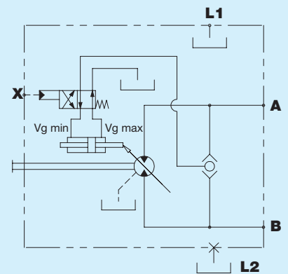
液压图
