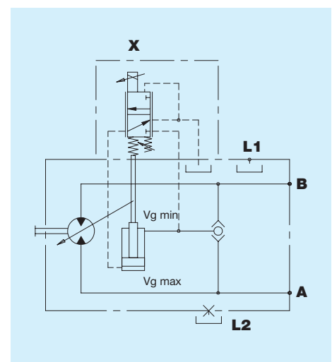
液压图
