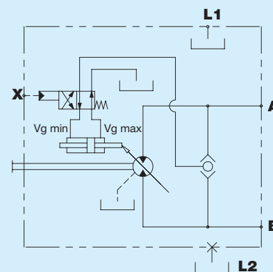
液压图
