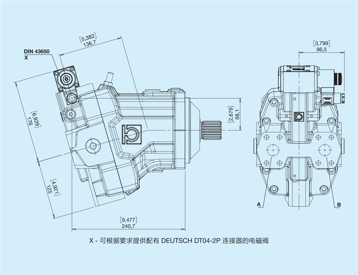
液压图
